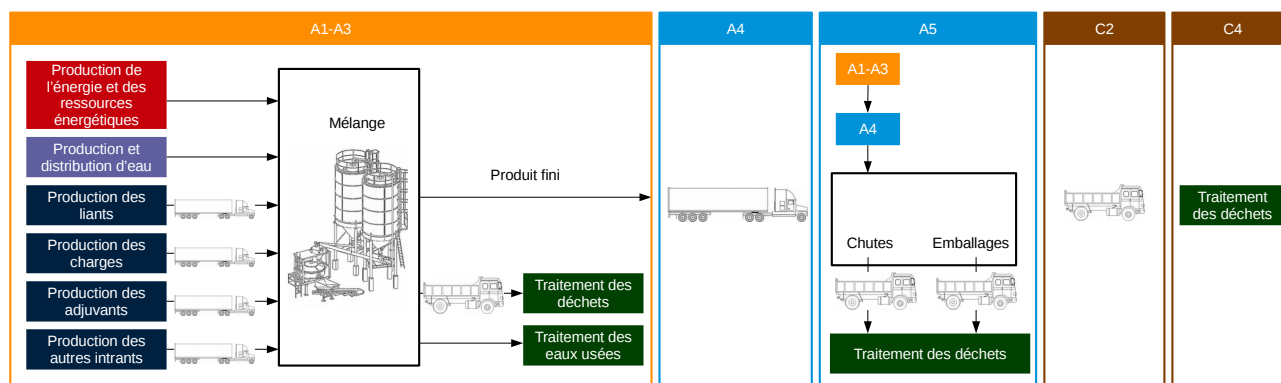
Figure 1 : Diagramme de flux et frontières du système
